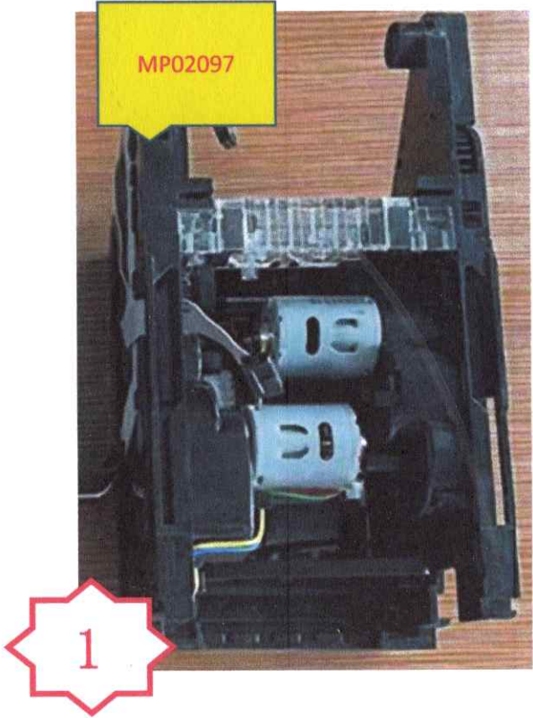
图一，按照物料清单折包材，每格放 1 个 MP02097，共 2 层 16 个
